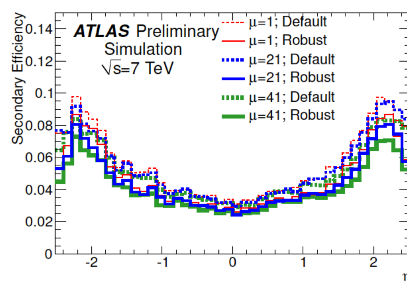
(d) Secondary efficiency vs \eta
